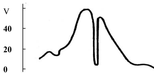
Рис.16. Скорость ветра при прохождении тайфуна через Манилу 20 октября 1882 г.
