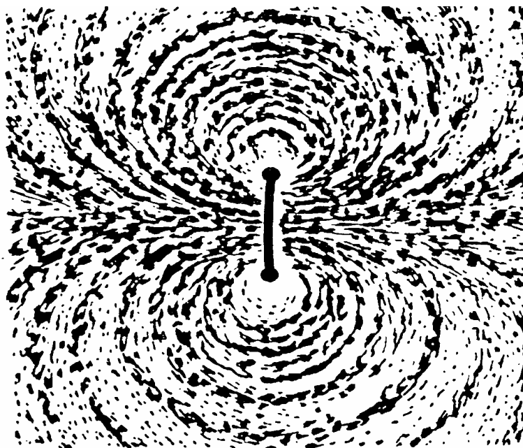
Рис.9. Силовые линии магнитного поля кругового тока, визуализированные при помощи порошка железа.
