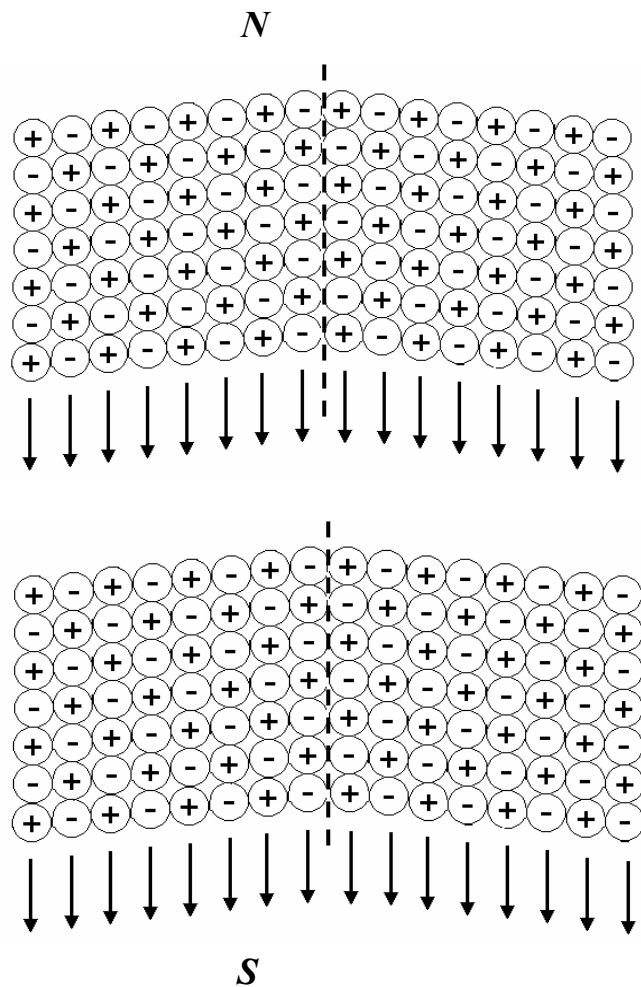
Рис.19. Однородное магнитное поле, возбуждаемое двумя магнитами (круговыми токами) в эфирной среде. Магниты повернуты разноименными полюсами навстречу друг другу.
