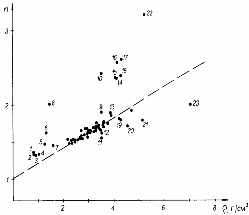
Рис.11. Зависимость между коэффициентом преломления n и плотностью \rho некоторых жидких и твердых веществ, минералов (Составлено по данным [56, 57]).
