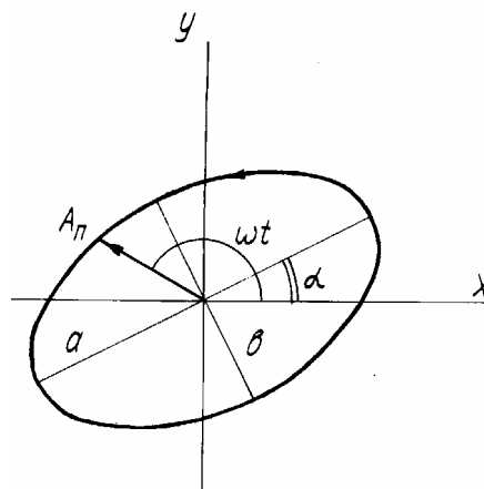
Рис.3. Эллиптическая форма смещения частиц среды в твердом теле при распространении сдвиговых волн [38].
