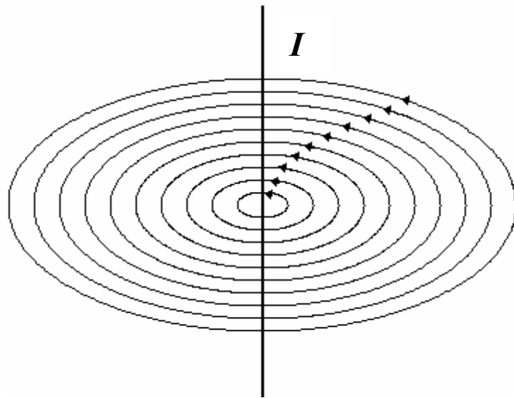
Рис.15. Эквипотенциальные линии магнитного поля в эфирной среде (вакууме) вокруг линейного проводника с током I .
