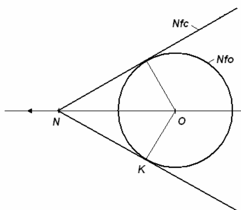
Рис. 23. Образование фронта электромагнитной волны от источника, движущегося со скоростью V , превышающей скорость света C .
