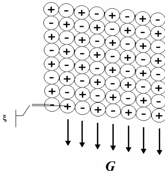
Рис.18. Однородная деформация эфирной среды вблизи сильного магнита или соленоида с током. Пример постоянного градиента напряженности поля в поперечном направлении к силовым линиям. Подобный градиент можно наблюдать в средней части очень длинного соленоида (магнита).
