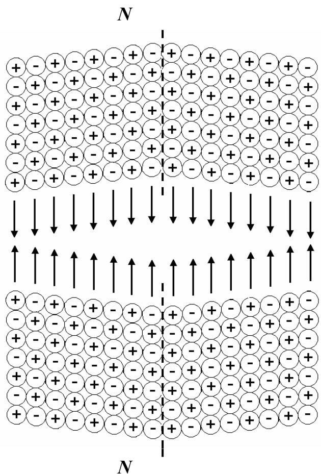
Рис.20. Однородное магнитное поле, возбуждаемое двумя магнитами (круговыми токами) в эфирной среде. Магниты повернуты одноименными полюсами навстречу друг другу
