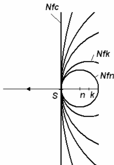
Рис. 22. Образование фронта электромагнитной волны от источника, движущегося со скоростью V равной скорости света C .
