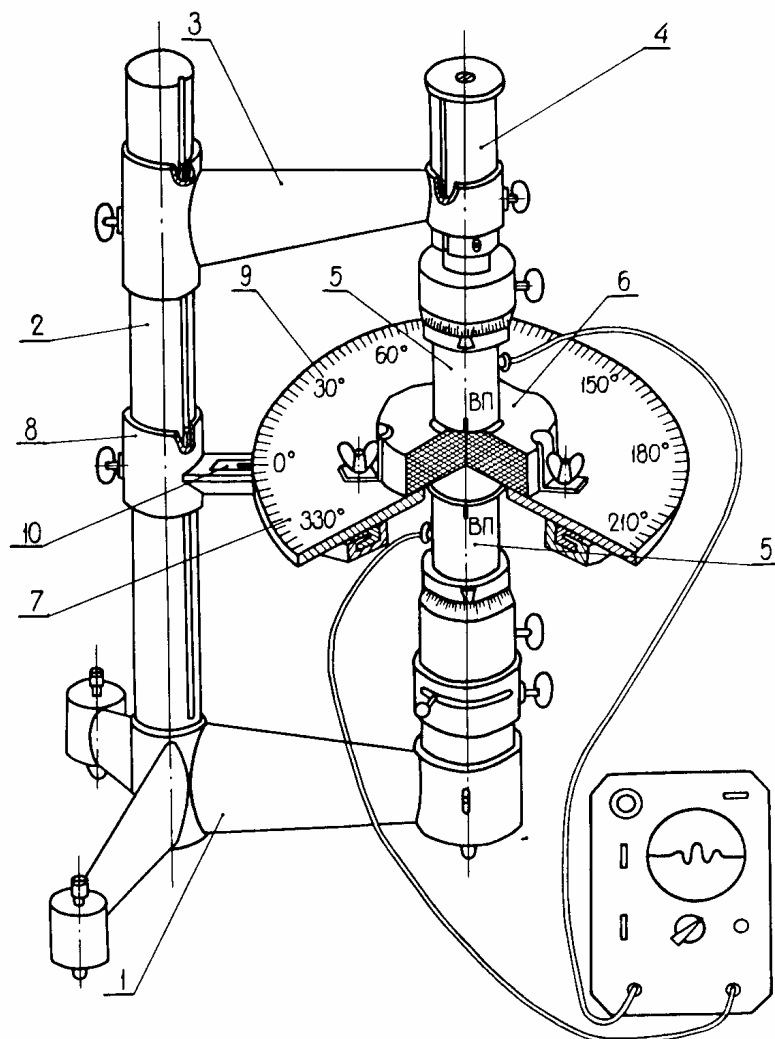
Рис.1. Конструкция акустополярископа с поворотной платформой. 1 - основание; 2 - стойка; 3 - кронштейн; 4 - подвижный шток; 5 - преобразователи; 6 - образец; 7 - поворотная платформа; 8 - дополнительный кронштейн; 9 - шкала углов; 10 - указатель.
