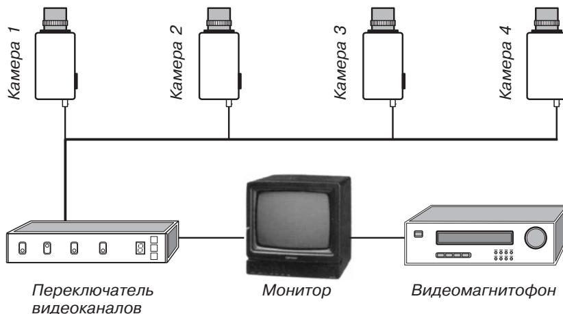
Рис. 4.7. Четырехкамерная система телевизионного наблюдения
