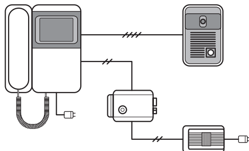
Рис. 4.5. Схема подключения домофона с электрическим замком
