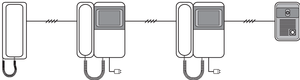
Рис. 4.6. Схема подключения двух домофонов к одной камере
