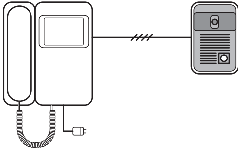
Рис. 4.4. Схема подключения домофона
