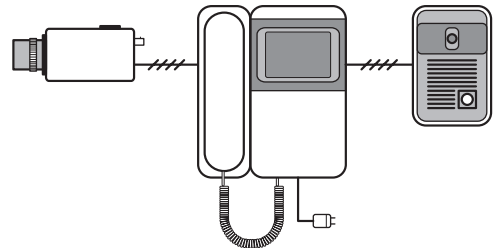
Рис. 4.3. Схема подключения двух камер и домофона
